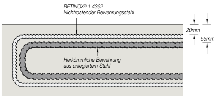
Mindestbetondeckung C_{nom} am Beispiel Expositionsklasse XD1
