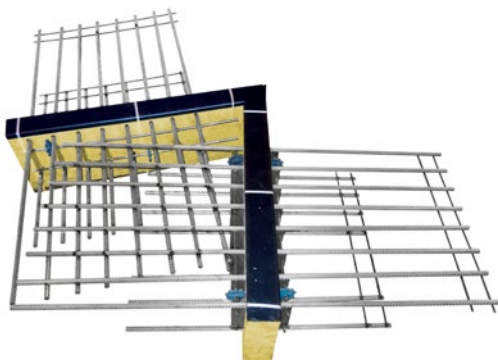
Eckelemente ungleich 90°
