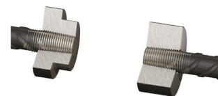
Ancon-TTH Endverankerung 1 Gewinde, 1 TTH Endverankerung montiert
