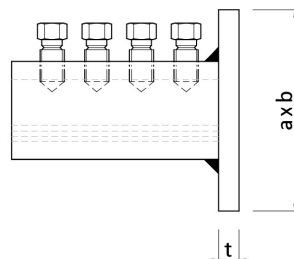
Ancon-MBT ET Tête d'ancrage
