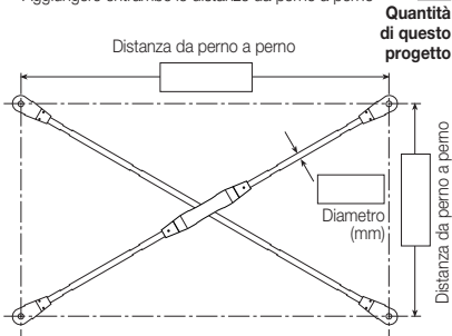
Giunzione a croce regolare con manicotto di giunto Aggiungere entrambe le distanze da perno a perno
