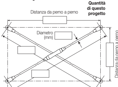
Giunzione a croce irregolare con manicotto di giunto
